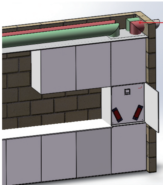
一体式外墙防风雨风帽
