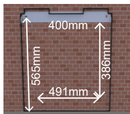
一体式外墙防风雨风帽
