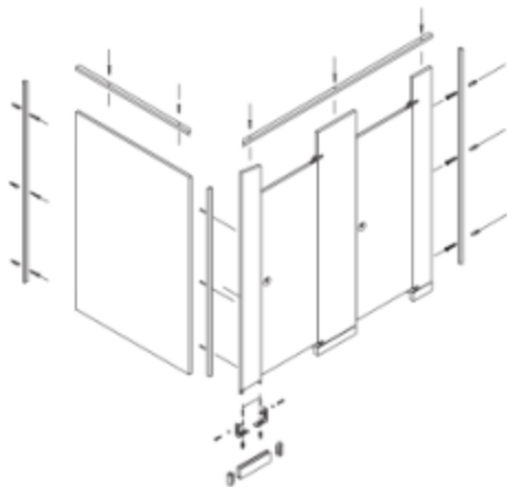
2: 立板与隔板之间“U”型槽安装方法
