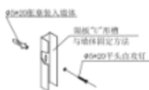
靠墙“U”型槽安装方法
