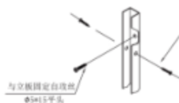
隔板安装方法
