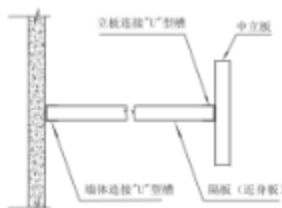
隔板安装方法
