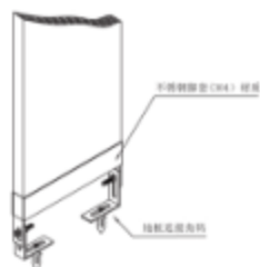
1: 立板安装方法
