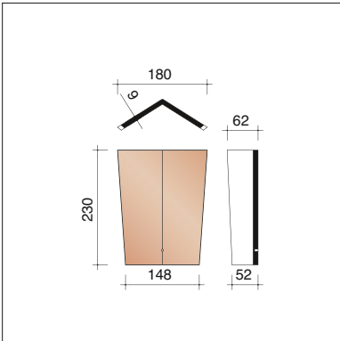
POOO3701 (6 stuks/lm) Kleine hoekige noordboom
