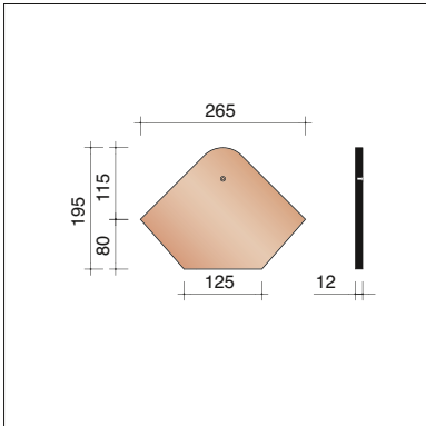
POOO2842 Kopplaat voor hoekige vorst zonder sluiting 45°
