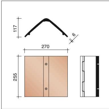
POOO2802 (4 stuks / lm) Hoekige vorst zonder sluiting 45°
