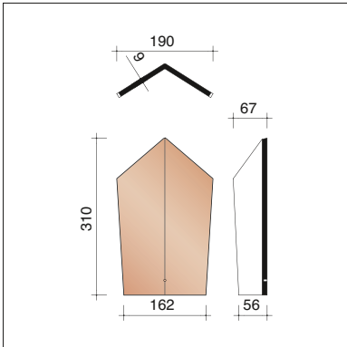
POOO3711 Kleine hoekige beginnoordboom
