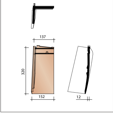
PELF7120 (3,6 stuks/lm) Speciale linker halve gevelpan
