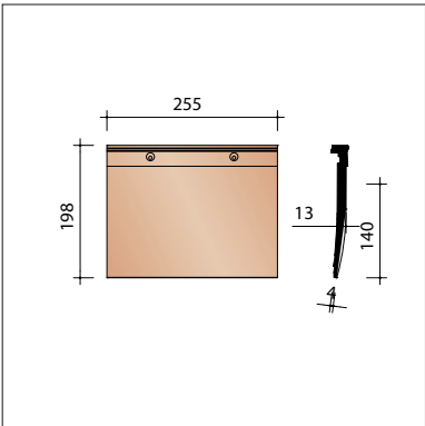
PELF8110 (4 stuks / lm) Korte pan
