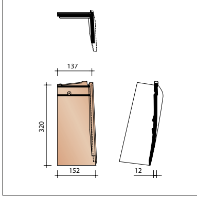
PELF7130 (3,6 stuks/lm) Speciale rechter halve gevelpan
