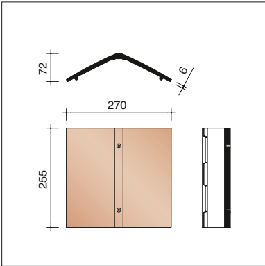
POOO2801 (4 stuks / lm) Hoekige vorst zonder sluiting 30°
