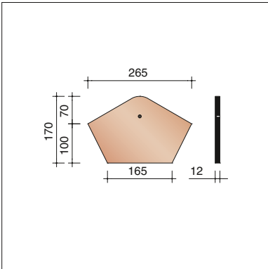
POOO2841 Kopplaat voor hoekige vorst zonder sluiting 30°
