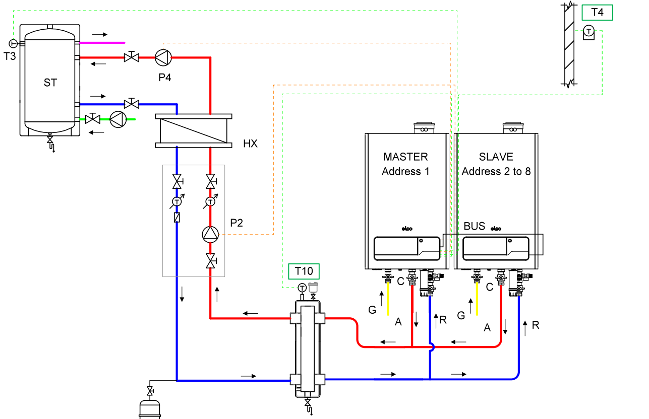
系统五 级联壁挂炉热水系统（板换间供）
