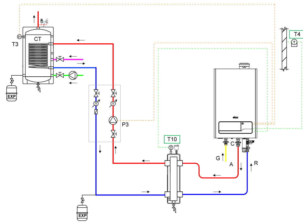
系统四 单台壁挂炉热水系统（间供）
