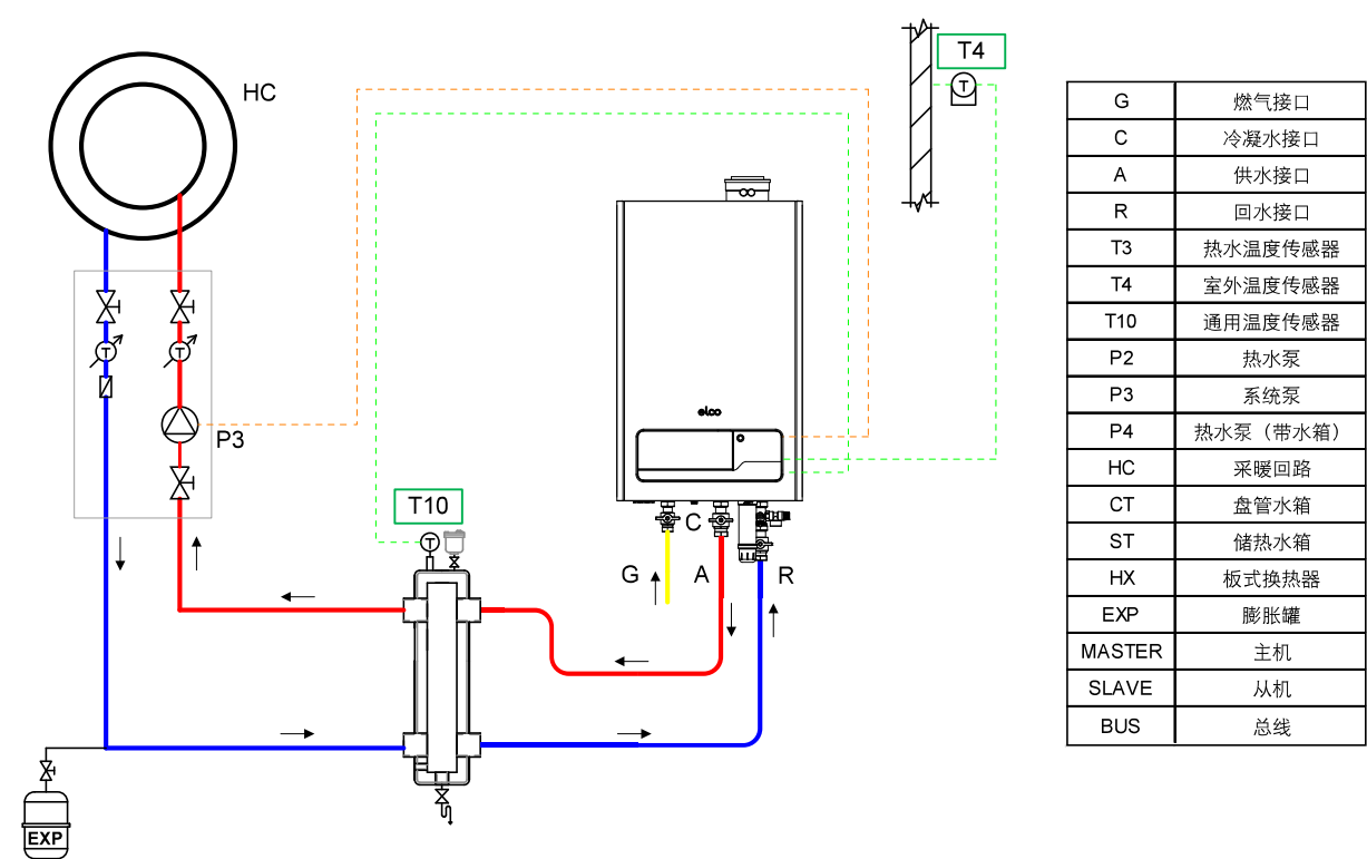
系统一 单台壁挂炉采暖系统（直供）
