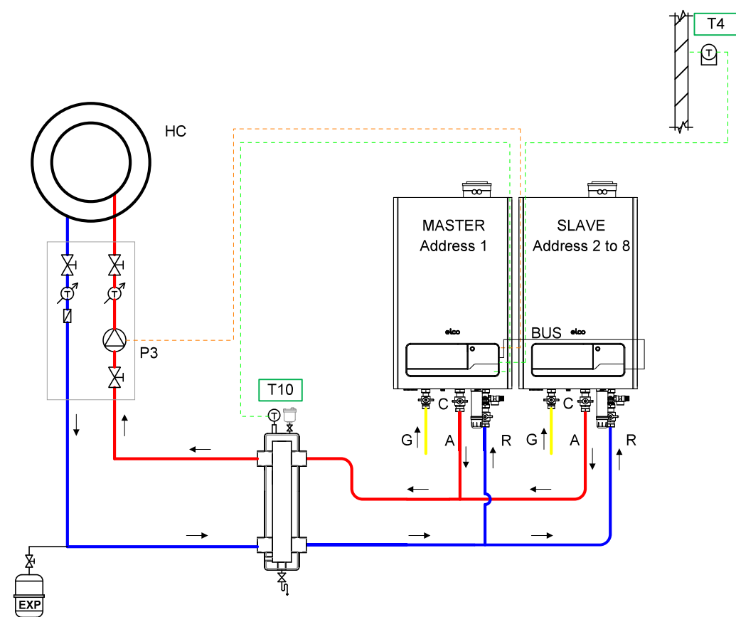
系统二 级联壁挂炉采暖系统（直供）
