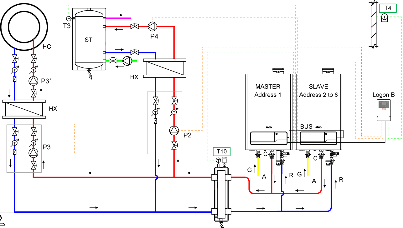
系统六 级联壁挂炉采暖+热水系统（板换间供）
