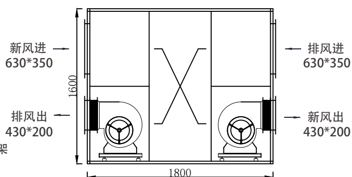
6000 风量新风机组工作原理图
