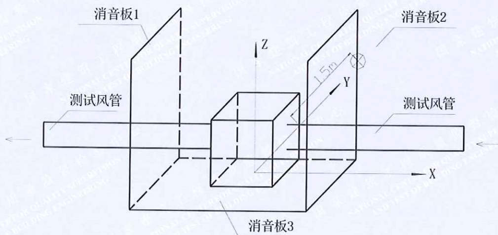
图 1 噪声测点布置图
